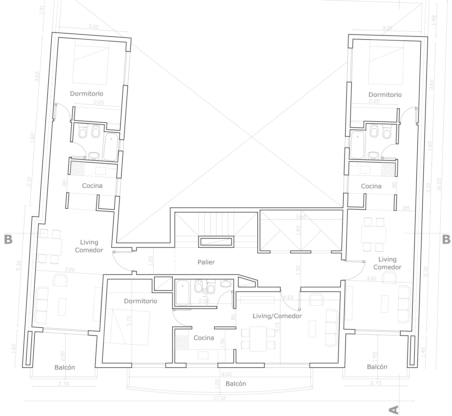
PLANTA TIPO
